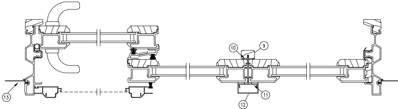
3 Panel Jamb Detail - XOO R
