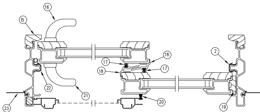
Jamb Detail - XO
