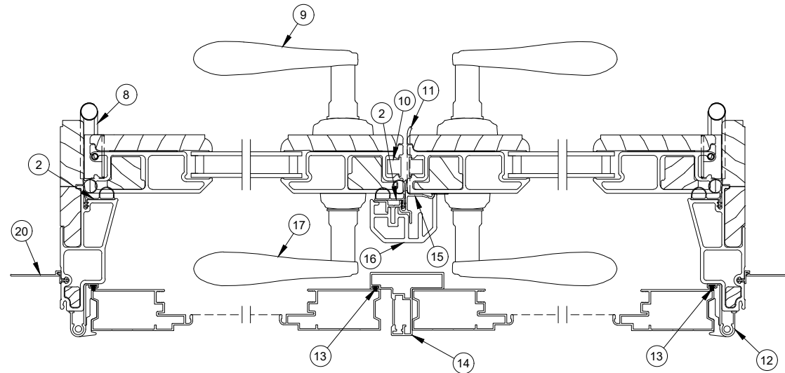
Jamb Detail
