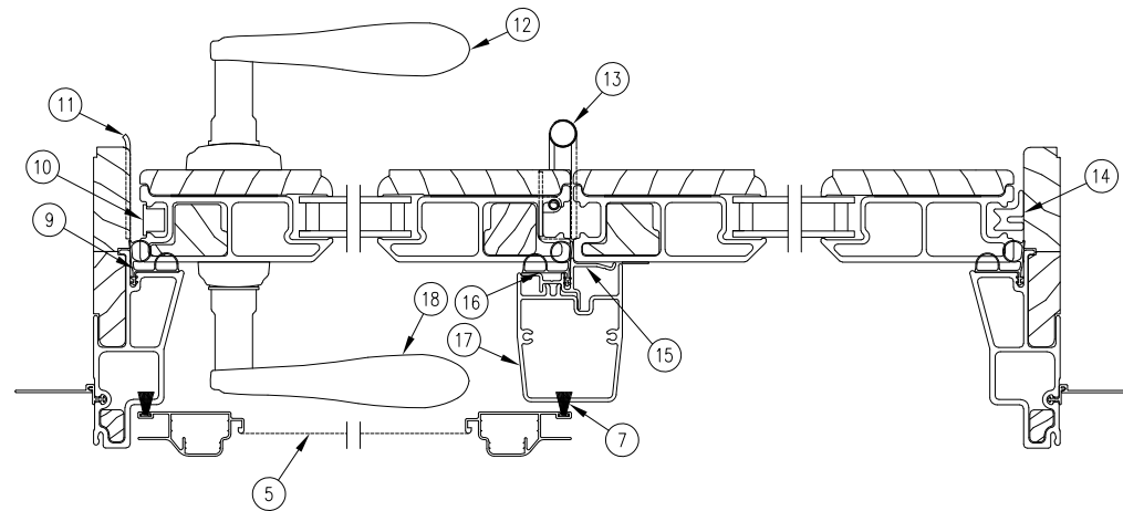
Jamb Detail
