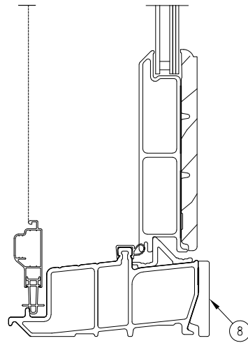
Sill Detail HP/IZ3
