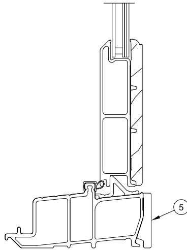
Sill Detail HP/IZ3
