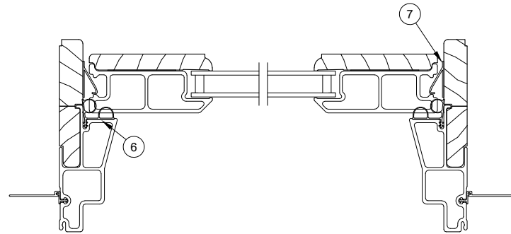
Jamb Detail
