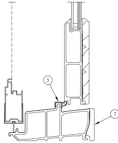
Sill Detail HP/IZ3
