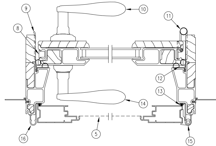
Jamb Detail
