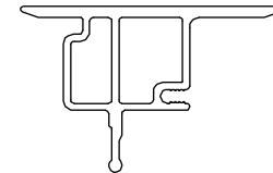
Exterior Astragal, A2997 OXXO
