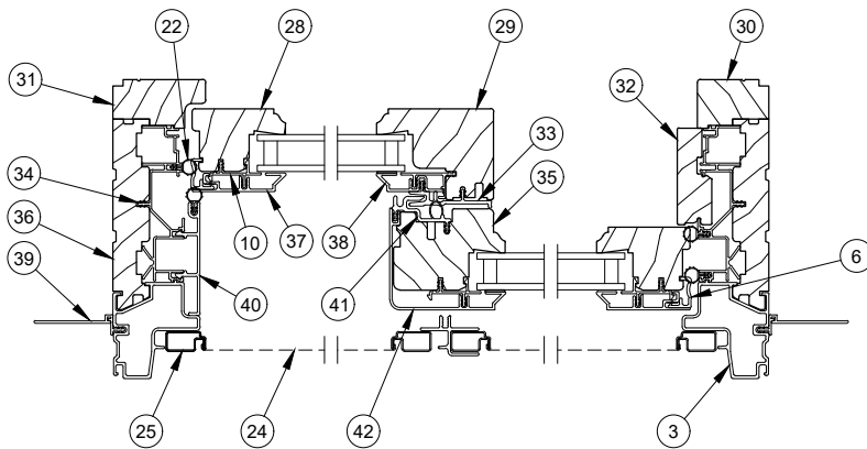
Jamb Detail
