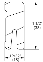
Sill Liner (oak), W2528
