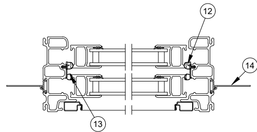
Jamb Detail
