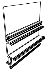
Nailing Fin Vertical, CMBC, V081
