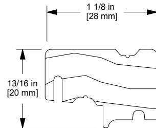
W13639 Astragal Base
